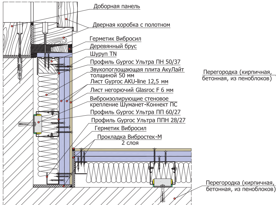
2.07.2 Примыкание облицовки стен к дверному проёму. Оформление внутреннего угла
