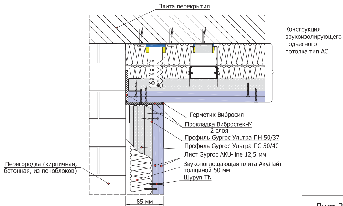
2.02.3 Примыкание облицовки стен к подвесному звукоизолирующему потолку
