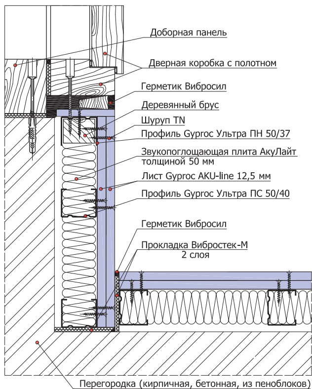
2.02.2 Примыкание облицовки стен к дверному проёму. Оформление внутреннего угла
