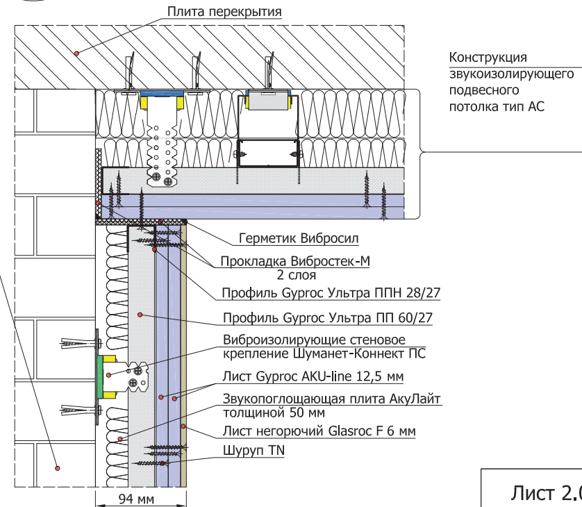
2.07.3 Примыкание облицовки стен к подвесному звукоизолирующему потолку
