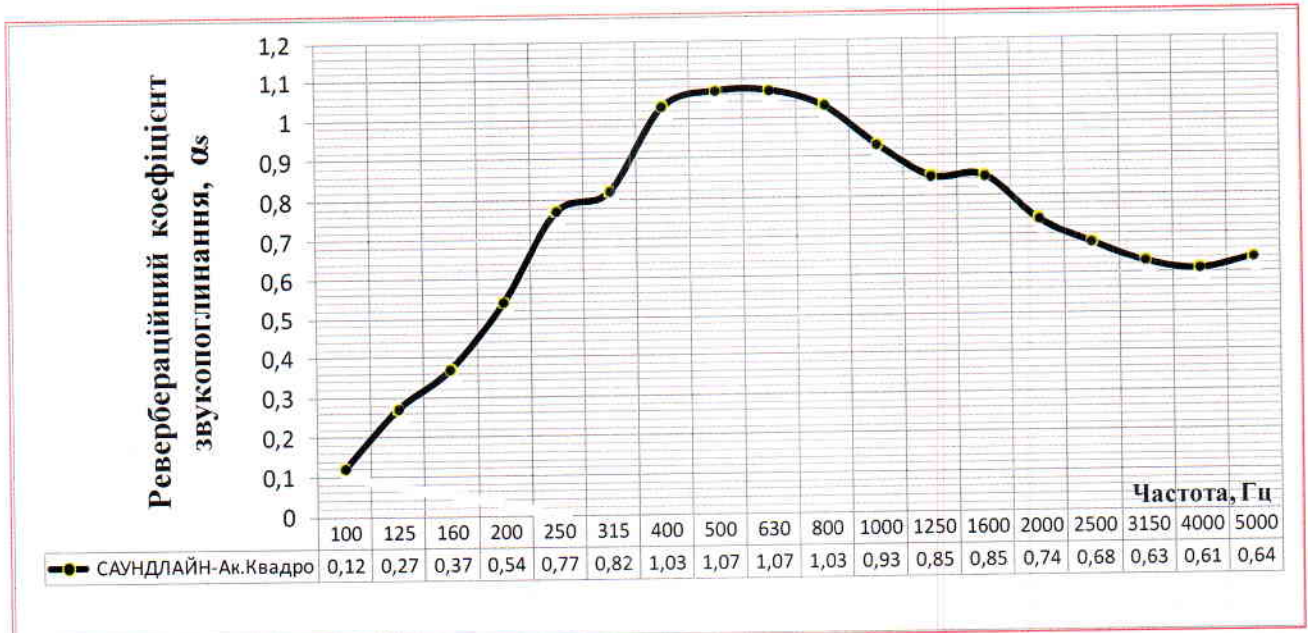
Рисунок 1 – Частотна характеристика ревербераційного коефіцієнта звукопоглинання ( \alpha_s ) звукопоглинальної конструкції «САУНДЛАЙН-Акустика Квадро», укладеної на жорсткій поверхні
